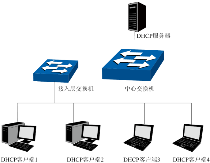
图 13-5 DHCP 网络典型应用
