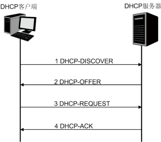
图 13-6 动态获取 IP 地址的过程
