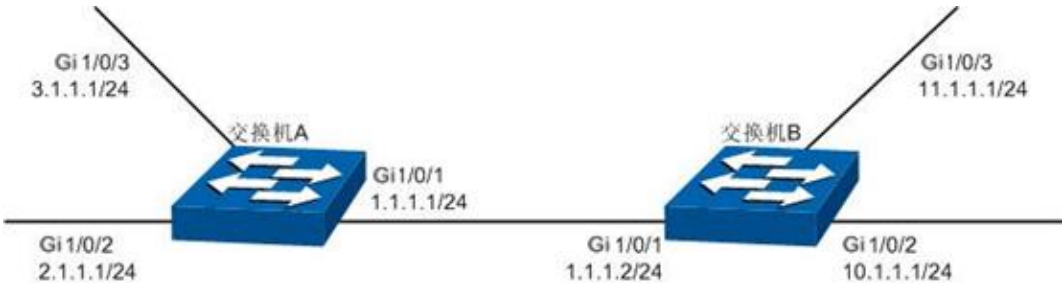
图 10-36 组网图
