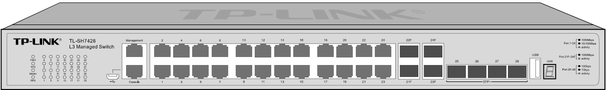
图 2-1 TL-SH7428 前面板
